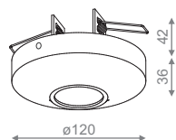
AQLED module / moduł AQLED
